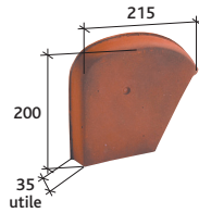
Fronton gauche pour faitière Shed Réf. 806 (5)
