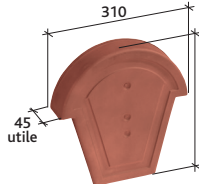
Fronton pour faitière 1/2 ronde à recouvrement Réf. 807
