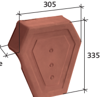
Fronton de rive universelle Réf. 1080 (5)
