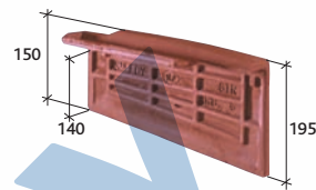
Okrajová taška pravá (4,5 ks/bm) Réf. 301.41
