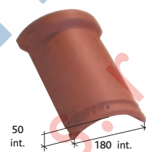
Hřebenáč malý (3 ks/bm) Réf. 700
