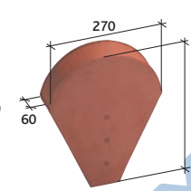
Ukončení hřebenáče malé Réf. 803
