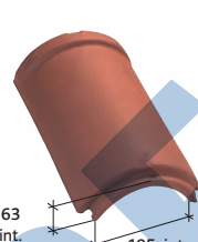
Hřebenáč (2,5 ks/bm) Réf. 702.
