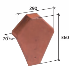
Ukončení hřebenáče univerzální Réf. 801
