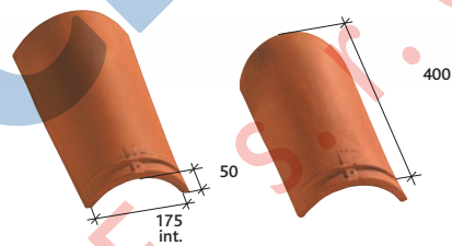
Hřebenáč kónický (2,5 ks / bm) Réf. 708
