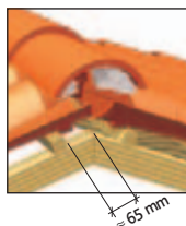
Hřeben v maltě
