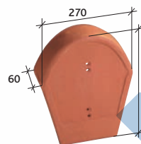
Uzávěr hřebene 90° Réf. 814
