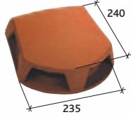
Klobouk prostupové tašky Ø 150 a Ø 120 Větrací otvor: 130 cm 2 Réf. 1000
