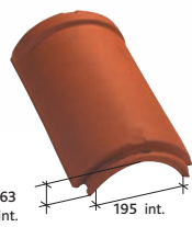
Hřebenáč (2,5 ks / bm) Réf. 702
