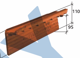
Okrajové tašky (levá, pravá) (2,5 ks / bm při laťování 400 mm) s krátkými klapkami Réf. 104.40RC et Réf. 104.41RC
