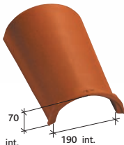
Hřebenáč kónický (2,5 ks / bm) Réf. 703
