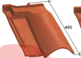
Hřebenová taška Réf. 104.100
