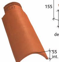
Poloviční taška Réf. 104.01
