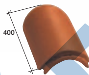
Koncový hřebenáč Réf. 851
